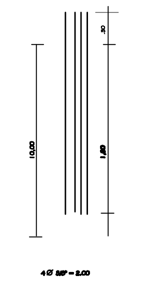
DET. DAS BROCAS b01 fck = 200cf cm2
