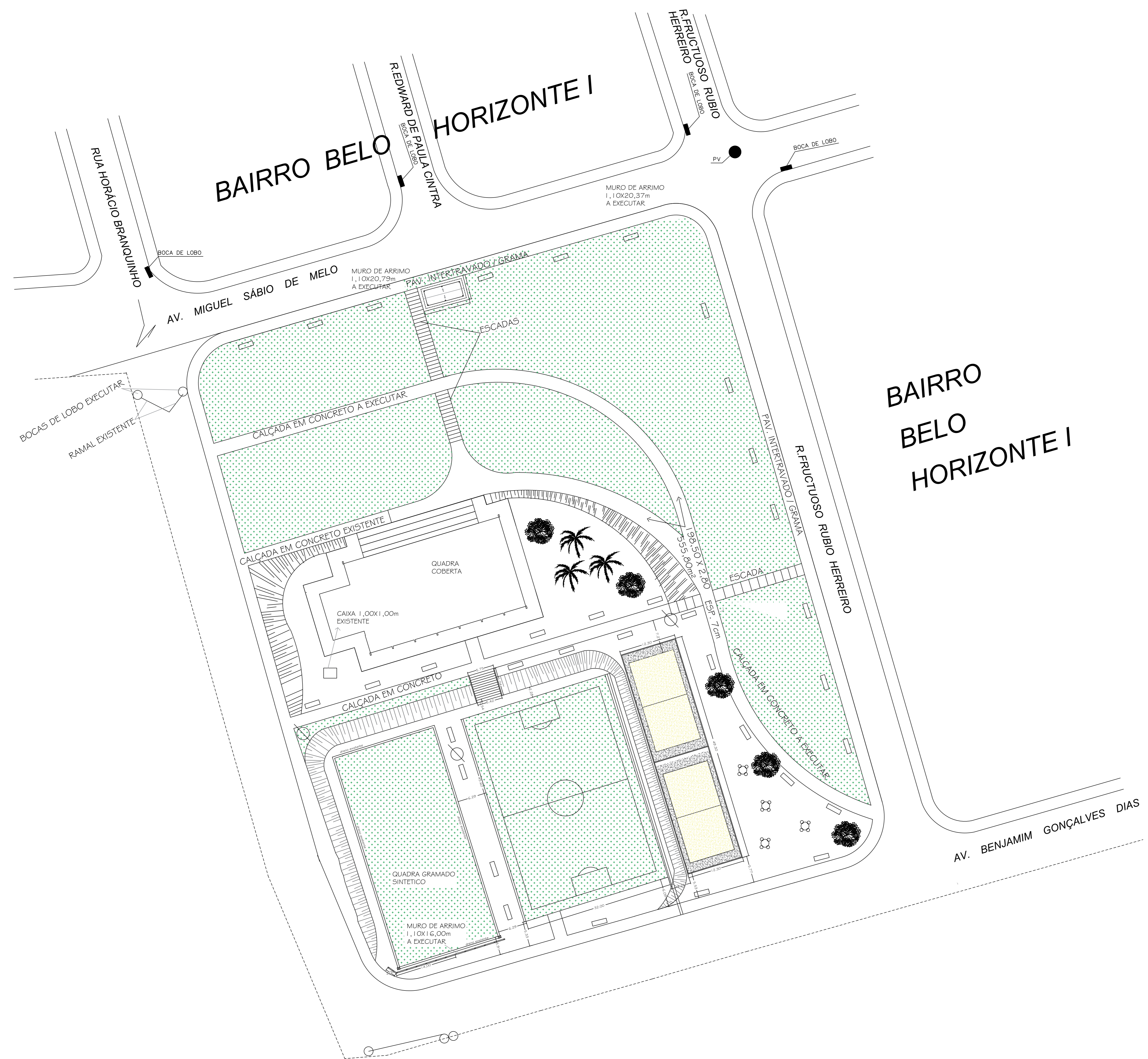
PLANTA DE LOCAÇÃO / IMPLANTAÇÃO
