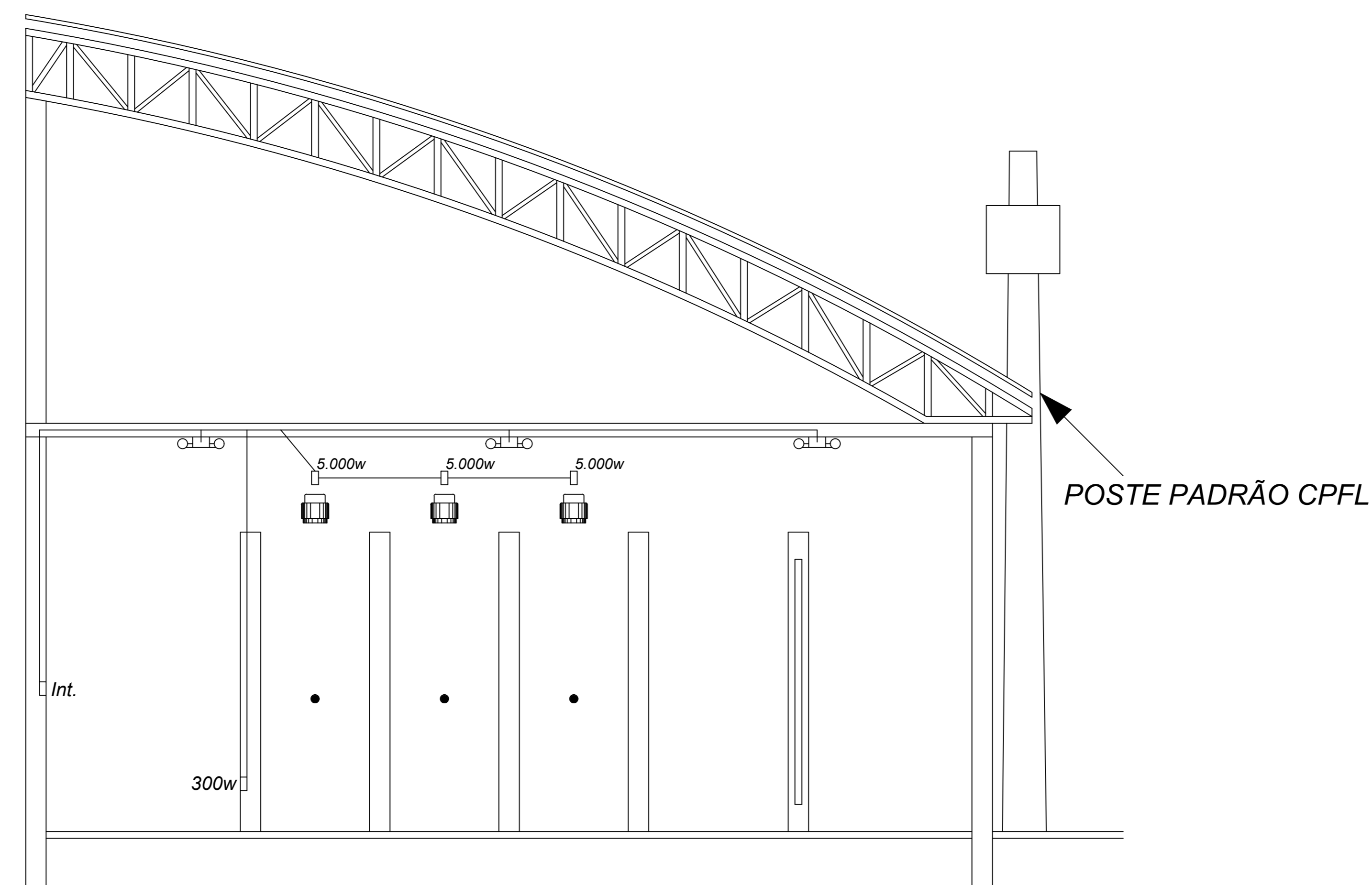
Corte Longitudinal - Elétrica esc. 1/50
